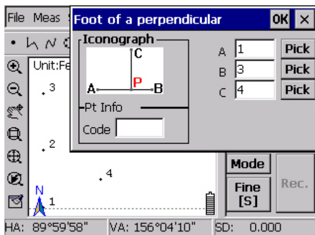
Основание перпендикуляра
