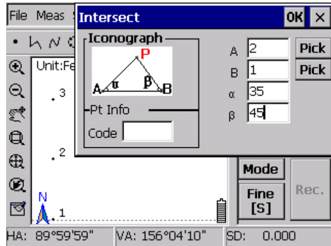
Прямое пересечение
