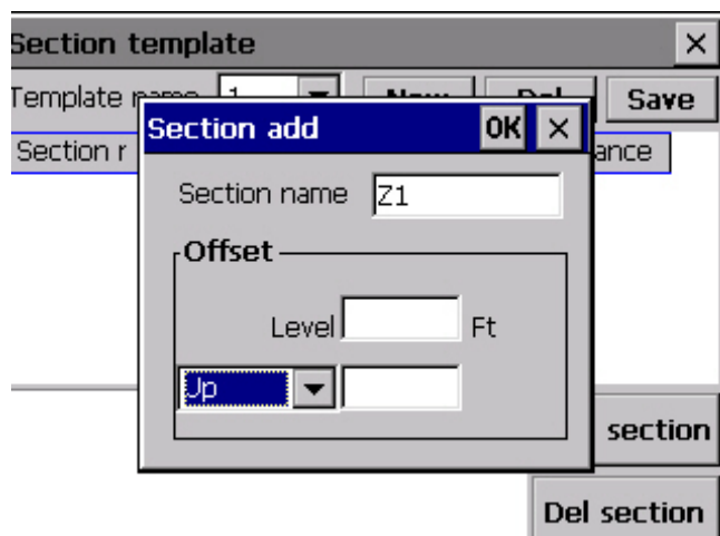
Добавление секции
