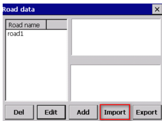
Импорт
