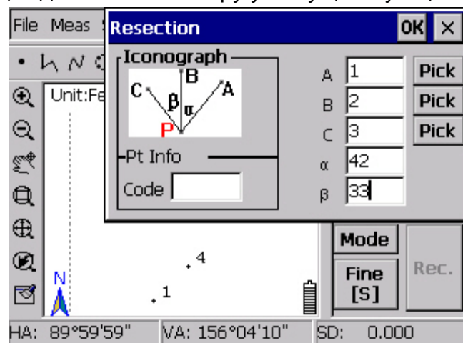
Обратная засечка
